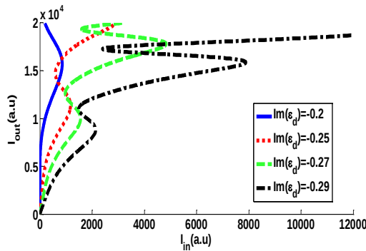
شکل ۶: منحنی شدت خروجی بلور فوتونی بر حسب شدت ورودی برای میزان بهره‌ی متفاوت -0.29 < \text{Im}(\epsilon_d) < -0.2 در حالت \theta = 10^\circ .
