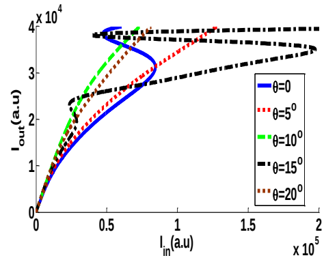
شکل ۴: منحنی شدت خروجی بلور فوتونی بر حسب شدت ورودی برای زاویه‌های ورودی مختلف \text{Im}(\epsilon_d) = 0 . در شکل ۵ منحنی شدت خروجی بلور فوتونی بر حسب شدت ورودی، برای میزان بهره‌ی متفاوت -0.15 < \text{Im}(\epsilon_d) < 0 در حالت \theta = 10^\circ ترسیم شده است.
