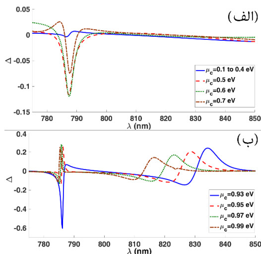
شکل ۲: طیف دایکرویزم دایروی برای فرود عمودی ( \theta=0^\circ ) یک موج قطبیده‌ی دایروی راستگرد و چپگرد به نانو ساختار طراحی شده به ازای انرژی‌های فرمی مختلف؛ (الف) در بازه‌ی ۰/۱ تا ۰/۷ الکترون ولت و (ب) در بازه‌ی ۰/۹۳ تا ۰/۹۹ الکترون ولت.
