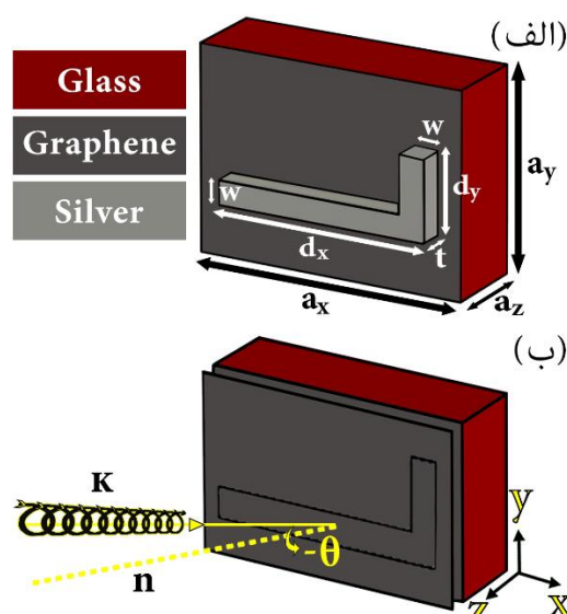
شکل ۱: طرح‌واره‌ای از سلول واحد نانو ساختار طراحی شده؛ (الف) یک نانومیله‌ی L شکل قرار گرفته بر روی تک لایه‌ی گرافن. (ب) نانومیله‌ی L شکل ساندویچ شده بین دو تک لایه‌ی گرافن.
