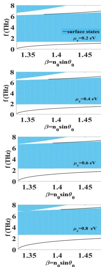
شکل ۳: منحنی پاشندگی بلور فوتونی و حالت‌های سطحی در پتانسیل‌های شیمیایی مختلف.
