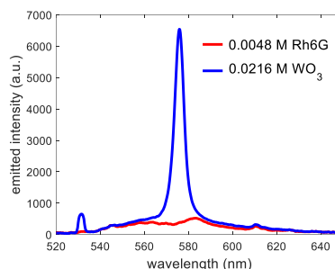
شکل ۵: طیف گسیل بر حسب طول موج به ازای انرژی دمشی ۴ میلی‌ژول بر ضریان برای محلول رنگدانه‌ی حاوی ذرات WO_3 (منحنی آبی) و فاقد آن‌ها (منحنی قرمز).
