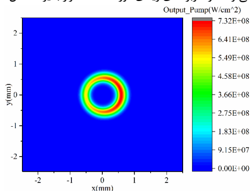
شکل ۴: نیمرخ لکه پمپ در انتهای بلور با اعمال تقویت غیرخطی
