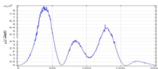
شکل ۷: تغییرات شار انرژی در داخل یک موجبر DLSPWs برحسب طول انتشار برای ساختاری که موجبر مشابهی در فاصله ۲۰۰ nm از آن قرار گرفته است
