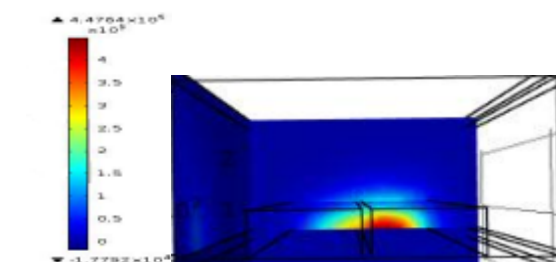
شکل ۱۱: توزیع شار انرژی در راستای y در طول 14600 \text{ nm} برای دو موجبر با مشخصات شکل (۸). شار انرژی در این طول انتشار ناقص‌تر به موجبر سمت راست منتقل شده است. در این ساختارها از بستر فلز استفاده می‌شود چون هرگاه از یک دی‌الکتریک استفاده کنیم، چه در حالت یک موجبر و چه در حالت دو موجبر، شار انرژی به سمت بستر موجبر هدایت می‌شود. در ساختار شبیه‌سازی زیر از
