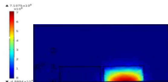
شکل ۸: توزیع شار انرژی در راستای y در طول 50 \text{ nm} برای دو موجبر با عرض 600 \text{ nm} و ضخامت 300 \text{ nm} و فاصله‌ی بین دو موجبر 50 \text{ nm} و طول موج نور فرودی 1.55 \mu\text{m} است.
