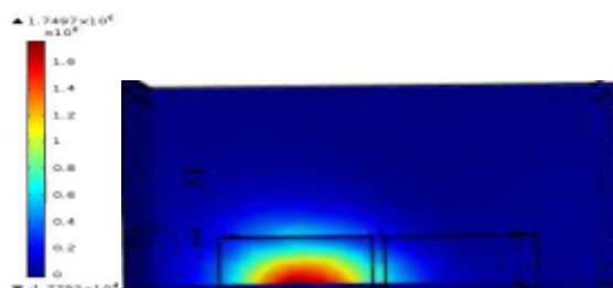
شکل ۱۰: توزیع شار انرژی در راستای y در طول 3000 \text{ nm} برای دو موجبر با مشخصات شکل (۸). شار انرژی در این طول انتشار ناقص به موجبر سمت چپ منتقل شده است.
