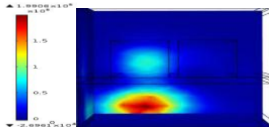
شکل ۱۲: توزیع شار انرژی در راستای y در طول 400 \text{ nm} برای دو موجبر با عرض و ضخامت 600 \text{ nm} و فاصله‌ی بین دو موجبر 100 \text{ nm} که طول موج نور فرودی 1.55 \mu\text{m} است.
