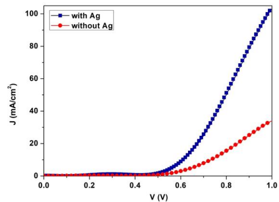
شکل ۵: منحنی مشخصه چگالی جریان- ولتاژ، با حضور نانوذرات پلاسmoniکی نقره و بدون حضور آن در تاریکی.
