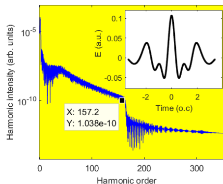
(شکل ۱) طیف هارمونیک برای میدان (درون شکل) با \tau_0 = 6 \text{ fs} و I = 1 \times 10^{14} \text{ W/cm}^2 , \lambda_0 = 800 \text{ nm}
