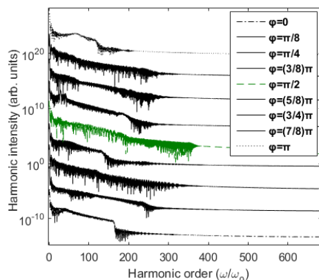
(شکل ۴) طیف هارمونیک برای فاز های مختلف با توجه به ثابت بودن کمیت های \lambda_1 = 1600 \text{ nm} , \lambda_0 = 800 \text{ nm} , R = 1 و \beta = 0.005 \text{phase} = 2\pi \frac{\Delta t}{T_1} = \omega_1 \Delta t \quad (9)
