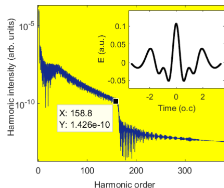
(شکل ۲) طیف هارمونیک برای میدان (درون شکل) با \tau_1 = 12 \text{ fs} و I = 1 \times 10^{14} \text{ W/cm}^2 , \lambda_1 = 1600 \text{ nm}
