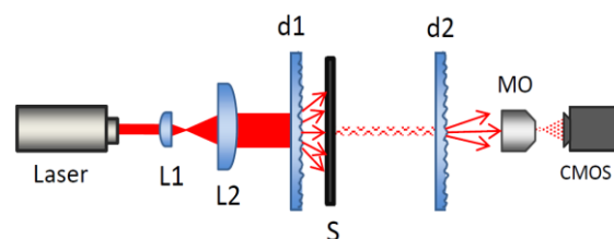
شکل ۱: چیدمان آزمایش.
