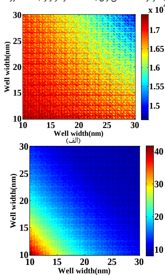
شکل ۳: (الف) بیشینه ضریب جذب و (ب) قله بسامد بر حسب ضخامت مواد \text{GaAs}_{0.7}\text{Al}_{0.3} و \text{GaAs} برای ۲۵ لایه و پتانسیل چاه -245.8\text{meV}
