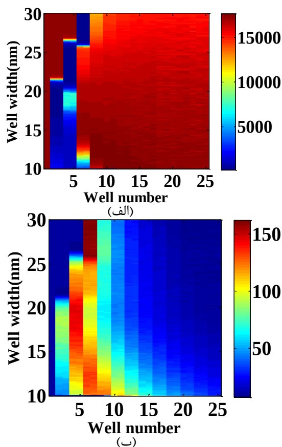
شکل ۴: (الف) بیشینه ضریب جذب و (ب) قله بسامد بر حسب ضخامت ماده \text{GaAs}_{0.7}\text{Al}_{0.3} و تعداد لایه‌ها، پتانسیل چاه -245.8\text{meV} و ضخامت ماده \text{GaAs} ۱۰ نانومتر.
