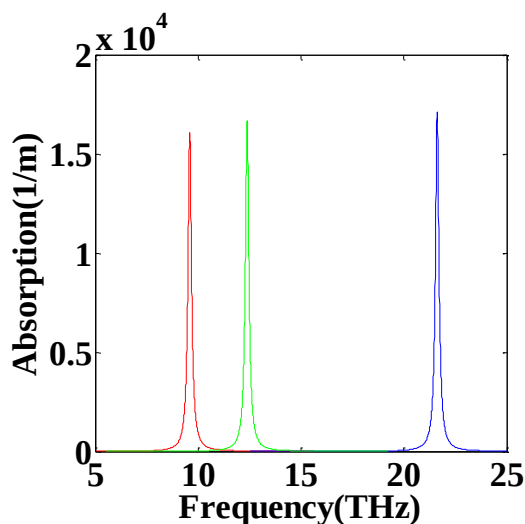
شکل (۲): طیف جذب به صورت تابعی از بسامد برای ۲۵ لایه برای منحنی قرمز ضخامت لایه فرد ۲۵nm ضخامت لایه زوج ۲۵nm ارتفاع ۲۴۵.۸mev. منحنی سبز برای ۲۰ لایه، ضخامت لایه فرد ۲۰nm ضخامت لایه زوج ۲۰nm ارتفاع ۲۴۵.۸mev و منحنی آبی برای ۲۵ لایه، ضخامت لایه فرد ۱۰nm ضخامت لایه زوج ۱۵nm ارتفاع ۲۴۵.۸mev
