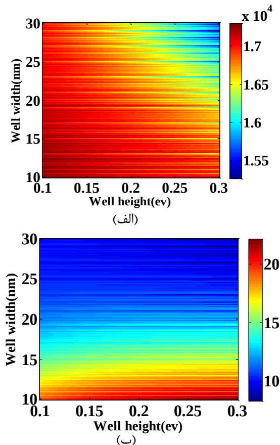
شکل ۵: (الف) بیشینه ضریب جذب و (ب) قله بسامد بر حسب ضخامت ماده \text{GaAs}_{0.7}\text{Al}_{0.3} و ارتفاع چاه پتانسیل برای 25 لایه.
