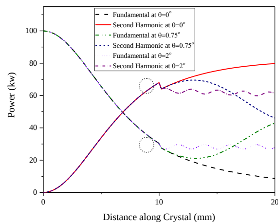
شکل ۳: تغییرات توان خروجی لیزر دمش و هماهنگ دومش در دوبار عبور از بلور KTP یک سانتی‌متری.
