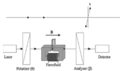
شکل ۱: چیدمان فارادی.
