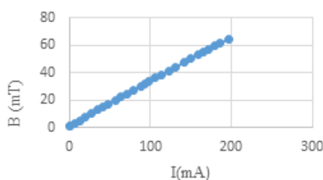
شکل ۵: تغییرات B بر حسب I.
