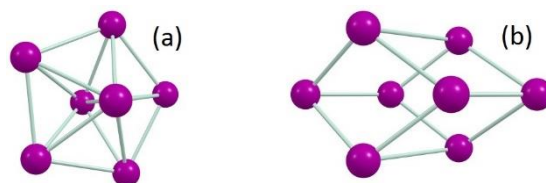
شکل ۱: ساختار نانوبلور (a) Si7 و (b) Ge7 که با روش DFT به حالت پایدار سراسری رسیده اند.
