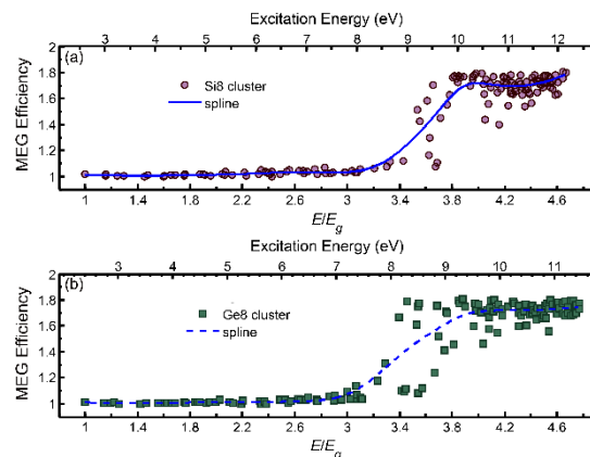
شکل 3: نرخ MEG برای Si8 (● با علامت (a) شکل) و Ge8 (□ (b) شکل). - - و - نمودار نرم شده نرخ MEG در Si8 و Ge8.
