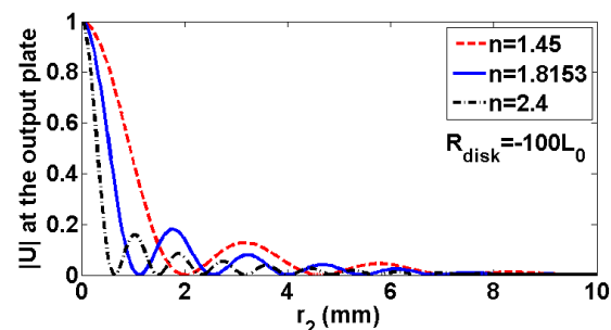
شکل ۲-ب: پروفایل عرضی باریکه در روی جفت‌ساز خروجی برحسب شعاع دیسک ( R_{disk} = -100L_0 ) و جفت‌ساز خروجی تخت است.
