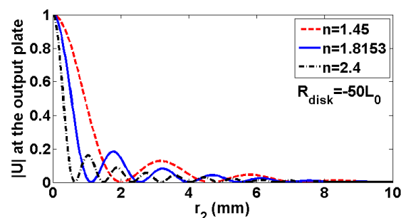
شکل ۲-الف: پروفایل عرضی باریکه در روی جفت‌ساز خروجی برحسب شعاع دیسک ( R_{disk} = -50L_0 ) و جفت‌ساز خروجی تخت است.
