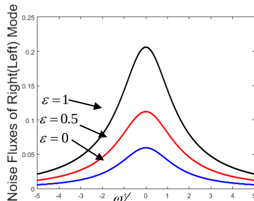
شکل ۱: نمودار شار نوفه مدراس (چپ) به ازای \varepsilon های مختلف
