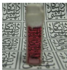
شکل ۲: کوت حاوی محلول رنگینه N719 که نمونه فوتو آند در آن قرار دارد.
