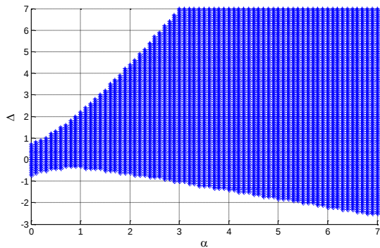
شکل (۳). ناحیه پارامتری وقوع دوپایایی برای شرایط مختلف نامیزانی بسامد کاواک با پرتو دمش ( \Delta ) نسبت به ضریب رشد پهنای خط ( \alpha ) در مقدار ثابت ( \mu=3 ).
