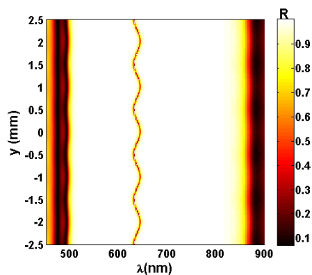
شکل ۳: طیف بازتابی از ساختار بر حسب فاصله عرضی y . ضریب شکست آنالیت n_{\text{Analyte}} = 1.33 و زاویه تابش ۶۵ درجه انتخاب شده است.
