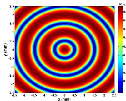
شکل ۴: نمودار بازتابندگی بر حسب تغییرات x و y ، که طول موج نور فرودی \lambda_0 = 632.8 \text{ nm} (لیزر هلیوم-نئون) و ضریب شکست آنالیت n_{\text{Analyte}} = 1.33 و زاویه تابش 65^\circ درجه انتخاب شده است.
