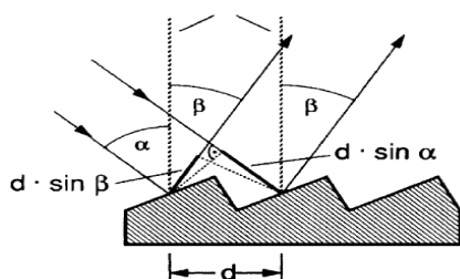
شکل ۱: پراش باریکه نوری از توری پراش
