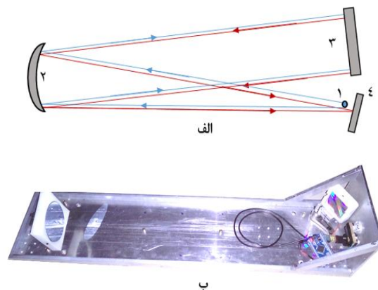
شکل ۳: الف) طرح اپتیکی طیف‌سنج (۱: روزنه ورودی باریکه- ۲: آینه مقعر با فاصله کانونی 70 \text{ cm} - ۳: توری پراش ۴: آشکارساز) ب) تصویر طیف‌سنج ساخته شده
