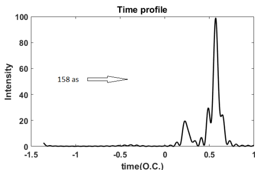
شکل ۲: پالس آتو ثانیه تولید شده توسط میدان لیزری سه رنگ
