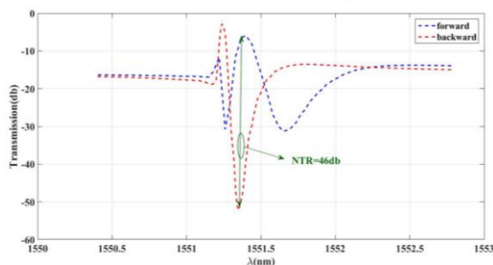
شکل ۴. طیف عبور رفت و برگشت برای ساختار شکل ۱ (ب) هنگامی که دامنه‌ی میدان الکتریکی ورودی 10^8 \times 1 V.m -1 است.
