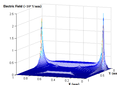
شکل ۶: شکل سه‌بعدی تغییرات میدان الکتریکی در مدل پیش یونش کرونا. محور عمودی مربوط به میدان الکتریکی ( \times 10^4 \text{ V/mm} ) است.
