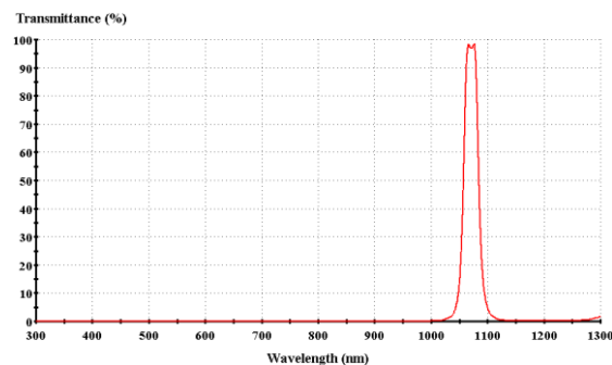
شکل ۳: طیف نهایی حاصل از طراحی دو فیلتر نوارگذر و بلندگذر بر روی دو سمت بستره‌ی جذبی RG850.
