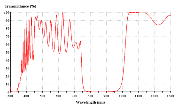
شکل ۲: طیف عبور حاصل از طراحی فیلتر بلندگذر بر روی بستره‌ی BK7.
