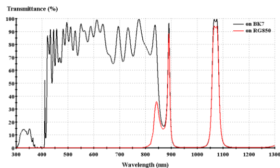
شکل ۱: طیف عبور حاصل از طراحی فیلتر نوارگذر باریک بر روی دو بستره‌ی BK7 و RG850.
