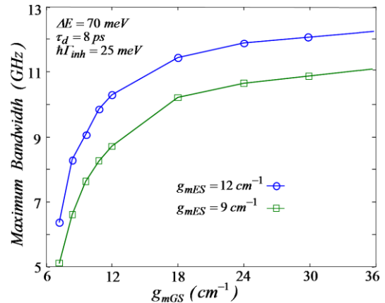
شکل ۷: ماکزیمم پهنای باند لیزر نقطه کوانتومی بر حسب ضریب بهره حالت پایه برای مقادیر متفاوت بهره حالت برانگیخته.
