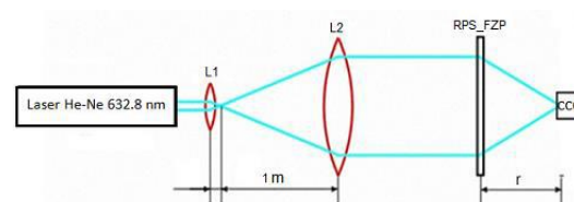
شکل ۳: چیدمان آزمایش
