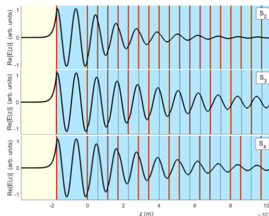
شکل ۳: توزیع میدان الکتریکی مد سطحی با فرکانس ۲ THz در سه مرتبه‌ی مولد مختلف
