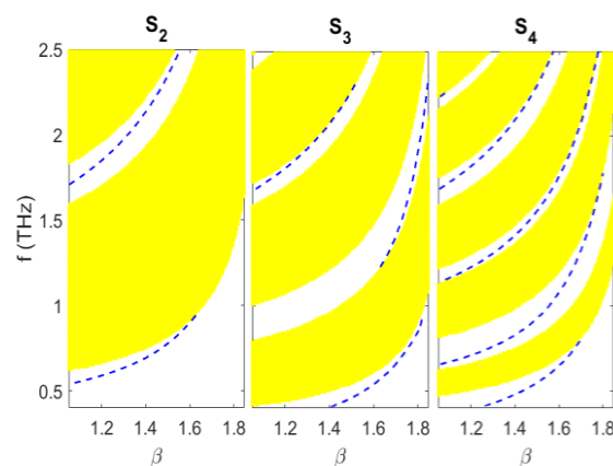
شکل ۲: منحنی‌های پاشندگی مدهای سطحی در فصل مشترک هوا و شبه بلور فوتونی به ازای مولدهای شبه متناوب فیبوناچی مرتبه‌های دو الی چهار.
