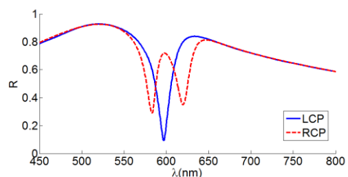
شکل ۳: طیف انعکاسی از ساختار طراحی شده برای قطبش‌های دایروی چپگرد و راستگرد.
