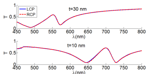
شکل ۶: طیف عبور از ساختار طراحی شده برای قطبش‌های دایروی چپگرد و راستگرد به ازای ضخامت‌های فراسطح با مقادیر ۳۰ و ۱۰ نانومتر.
