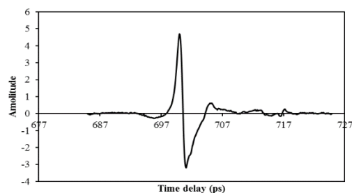
شکل ۳: سیگنال ترارترز پس از برهم‌کنش با نمونه گلوکز
