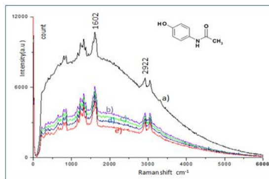
شکل ۲- طیف رامان قرص استامینوفن پس از (a) t=0 (b) t=20 ، (c) t=30 ، (d) t=40 و (e) t=60 دقیقه تاباندن نور لیزر به نمونه
