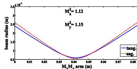
شکل ۶: کیفیت باریکه لیزر خروجی از چیدمان لیزر با طول بلور TGG برابر با ۱۲mm
