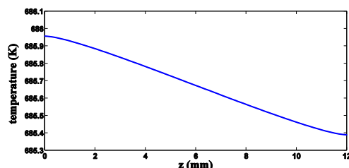
شکل ۴: توزیع دما در طول محور مرکزی بلور TGG
