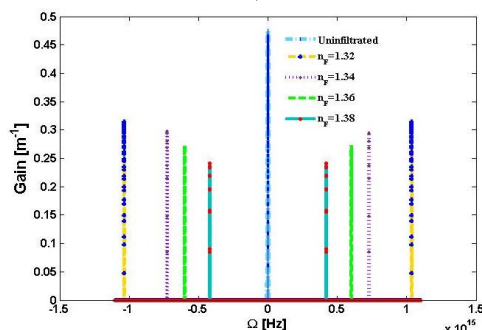
شکل ۴: نمودار تغییرات بهره بر حسب فرکانس در ناحیه پاشندگی عادی به ازای ضریب شکست‌های مختلف سیال نوری تزریق شده. طول PCF ۱۰ متر و توان پمپ 10 W انتخاب شده است.
