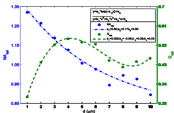
شکل ۳: منحنی آبی و منحنی سبز به ترتیب گشودگی عددی بهینه و بهینه راندمان تله‌ی نوری وارد شده بر حسب سایز میکروکره.
