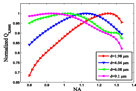
شکل ۲: راندمان تله‌ی نوری عرضی بهنجار شده بر حسب گشودگی عددی شیئی برای ۴ نوع سایز مختلف.
