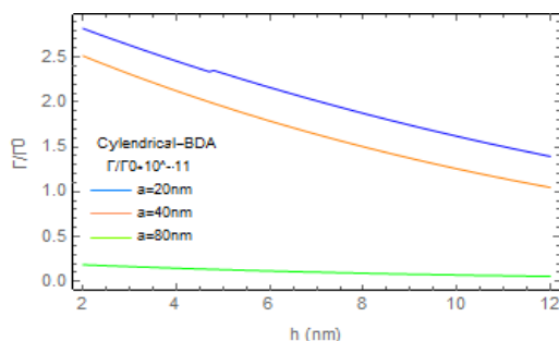
شکل ۳: تغییرات آهنگ گسیل خودبه‌خود نقطه‌ای کوانتومی در مجاورت استوانه‌ای طویل فلزی نسبت به فضای همگن بر حسب فواصل مختلف h
