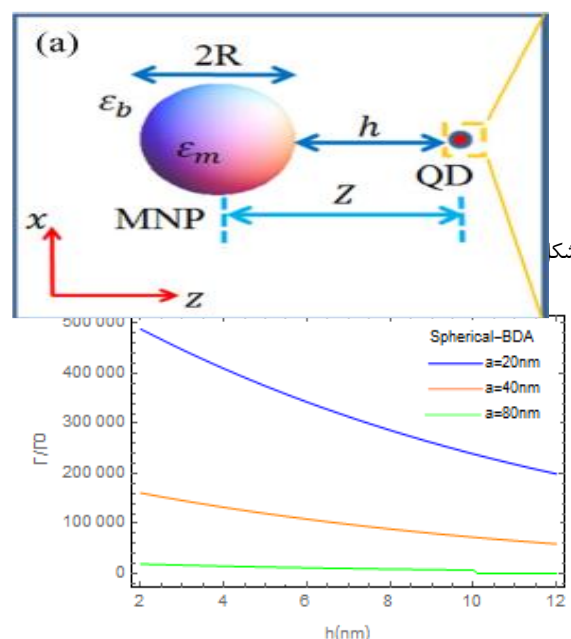
شکل ۲: تغییرات آهنگ گسیل خودبه‌خود نقطه‌ای کوانتومی در مجاورت نانوکره‌ی فلزی نسبت به فضای همگن بر حسب فواصل مختلف h
