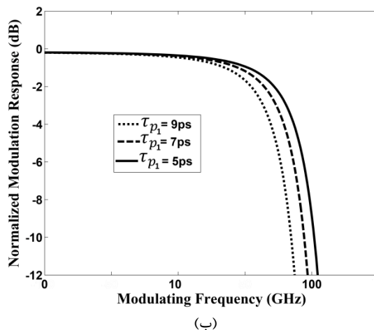
شکل (۳): پاسخ فرکانسی لیزر QC دو طول‌موجی در حالت (الف) برای تابش با طول‌موج \lambda_2 = 8.5 \mu\text{m} حالت (ب) برای تابش با طول‌موج \lambda_1 = 10.5 \mu\text{m}
