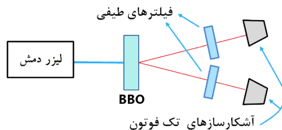
شکل ۱: طرح‌واره چیدمان تولید و آشکارسازی زوج فوتون‌های درهمتنیده‌ی حاصل از فرایند SPDC
