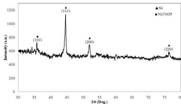
شکل ۳. الگوی پراش اشعه ایکس از ماده حاصل از کدنگی آلیاژ پایه نایتینول. ▲ پراش از صفحات فاز نیکل و ■ پراش اشعه ایکس از فاز Ni_3TiO_5 .
