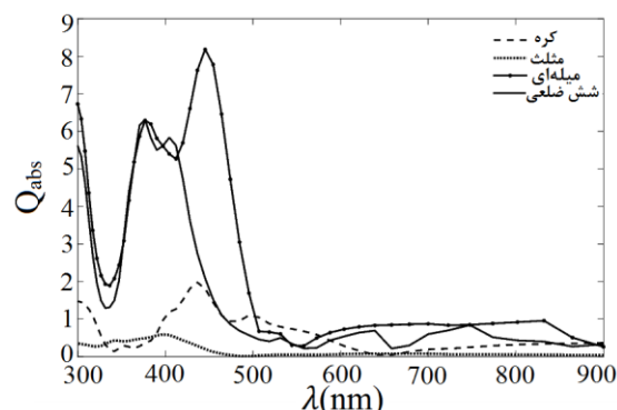
شکل ۶: نمودار Q_{abs} بر حسب طول موج برای نانوذرات کروی به قطر ۱۵۰ نانومتر، مکثی به ابعاد ۱۵۰ نانومتر، میله و شش ضلعی به قطر ۱۰۰ نانومتر و به ترتیب به ارتفاع ۵۰۰ و ۲۰۰ نانومتر از جنس نقره.
