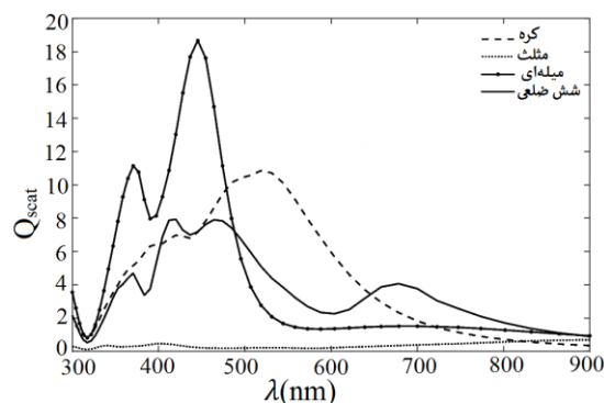
شکل ۴: نمودار Q_{sca} بر حسب طول موج برای نانوذرات کروی به قطر ۱۵۰ نانومتر، مکثی به ابعاد ۱۵۰ نانومتر، میله و شش ضلعی به قطر ۱۰۰ نانومتر و به ترتیب به ارتفاع ۵۰۰ و ۲۰۰ نانومتر از جنس نقره.
