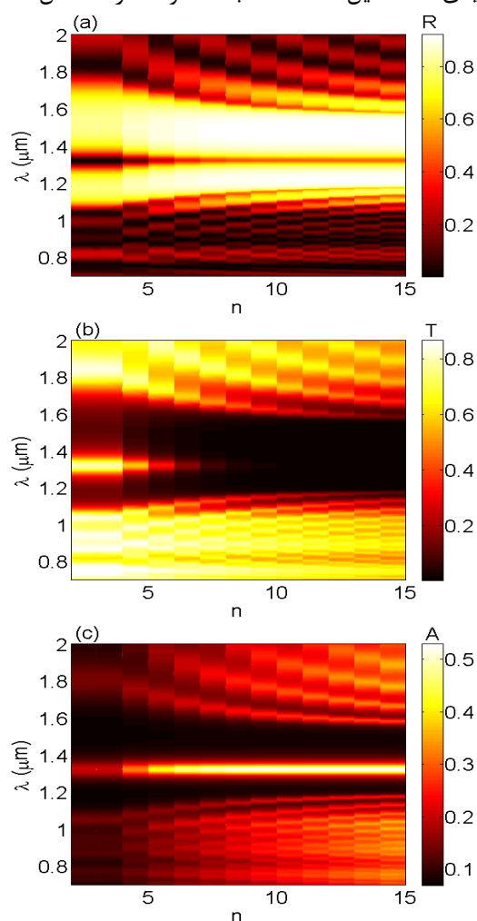
شکل ۲: طیف بازتابندگی (a)، تراگسیلندگی (b) و جذب (c) در صفحه‌ی n-\lambda برای m=3 . در اینجا T = 20^{\circ}\text{C} و \mu_c = 0.2\text{ eV} می‌باشند.
