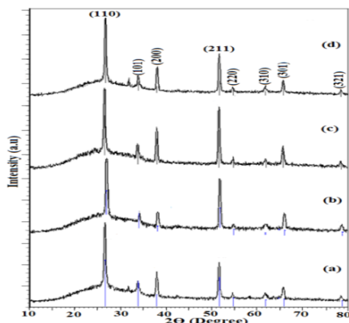
شکل ۱: طیف های XRD لایه های \text{SnO}_2 بازپخت شده در دماهای (a) بدون بازپخت، (b) 450^{\circ}\text{C} ، (c) 550^{\circ}\text{C} ، (d) 650^{\circ}\text{C}
