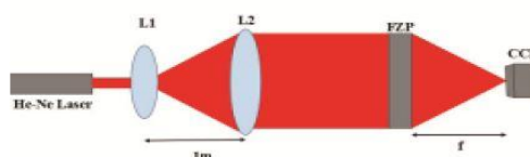
شکل ۵: چیدمان آزمایشگاهی
