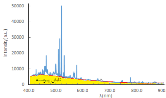
شکل ۲: طیف پلاسمای تولید شده از مس در فرآیند شکست اپتیکی با شدت لیزر 5/21 \text{ Gw/cm}^2 .
