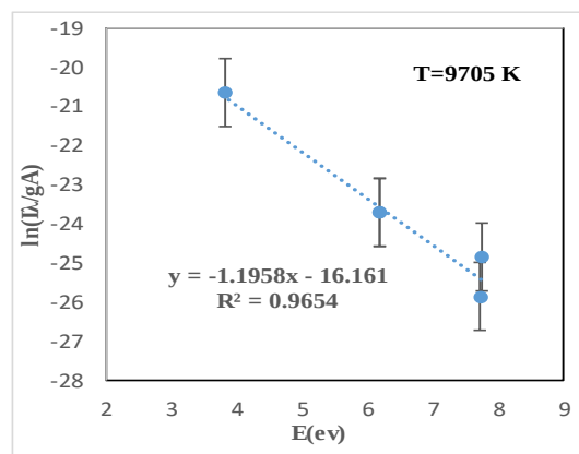
شکل ۳: نمودار بولتزمن خطوط Cu I برای تعیین دما.
