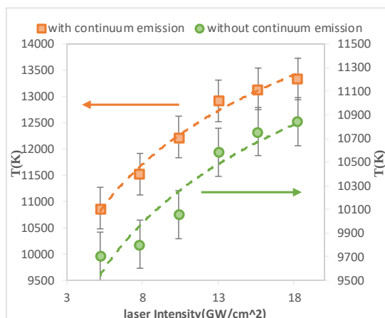
شکل ۴: مقایسه روند تغییرات دمای الکترون برای دو حالت: در نظر گرفتن تابش پیوسته (نقاط مربعی) و با کاستن آن از طیف (نقاط دایره‌ای) به انرژی لیزر با روش بولتزمن.
