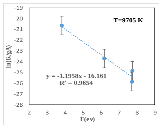
شکل ۵: نمودار بولتزمن خطوط Cu I برای تعیین دما.
