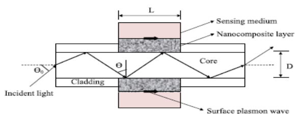
شکل ۱: شماتیک از سنسور فیبر نوری SPR
