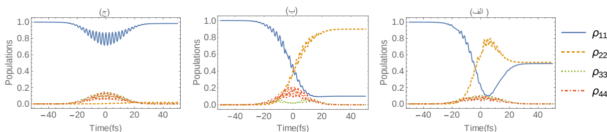
شکل ۲: تحول زمانی جمعیت‌ها برای \Phi = 0 (الف)، \Phi = \pi/2 (ب) و \Phi = \pi (ج). سایر پارامترهای استفاده شده عبارتند از: g_0 = 0.8 \text{ rad/fs} ، \nu = 100 \text{ m/s} و \Delta_{31} = \Delta_{42} = \Delta_{32} = -1
