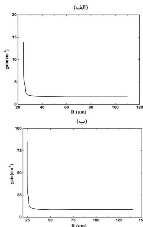
شکل ۵: ضریب بهره نسبت به فاصله از سطح هدف برای یون ژرمانیوم شبه نئون (الف) و \Delta t = 150 \text{ ps} (ب) و \Delta t = 100 \text{ ps} .
