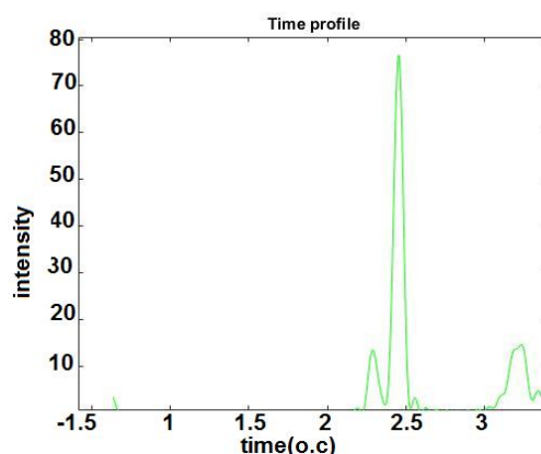
شکل ۶: پالس لیزر سه رنگی بدون چیرپ - ۱۵۸ آتوثانیه
