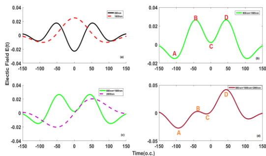
شکل ۱: (a) ترکیب دو میدان تک رنگ \lambda = 800 و \lambda = 1600 (nm) (b) ترکیب دو میدان دو رنگ و \lambda = 800 + 1600 (nm) (c) ترکیب دو میدان سه رنگی تک رنگ \lambda = 2000 (nm) (d) ترکیب دو میدان سه رنگی \lambda = 800 + 1600 + 2000 (nm)
